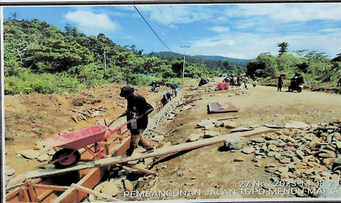
Pekerjaan pemasangan batu dengan mortar
