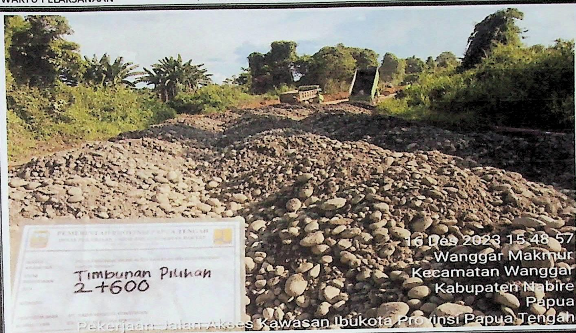
TIMBUNAN PILIHAN
