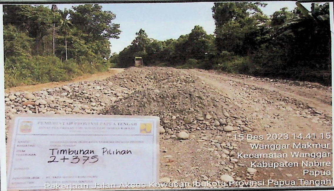
TIMBUNAN PILIHAN
