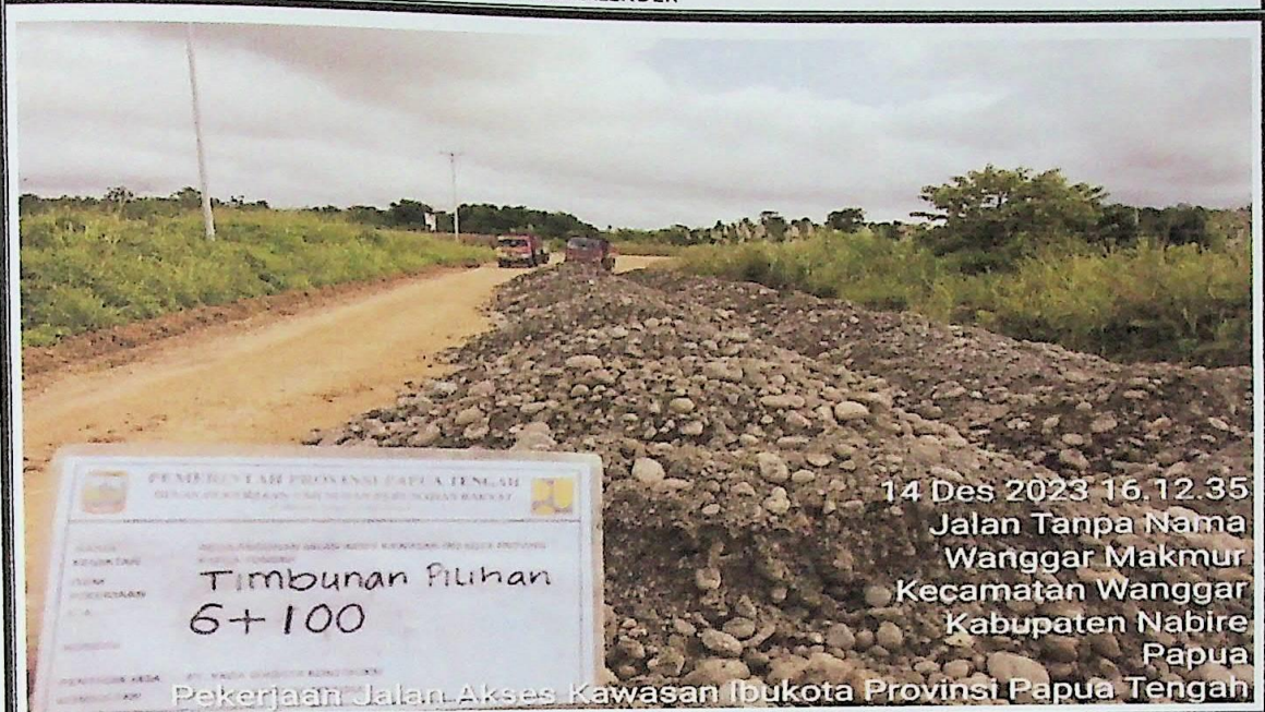
TIMBUNAN PILIHAN
