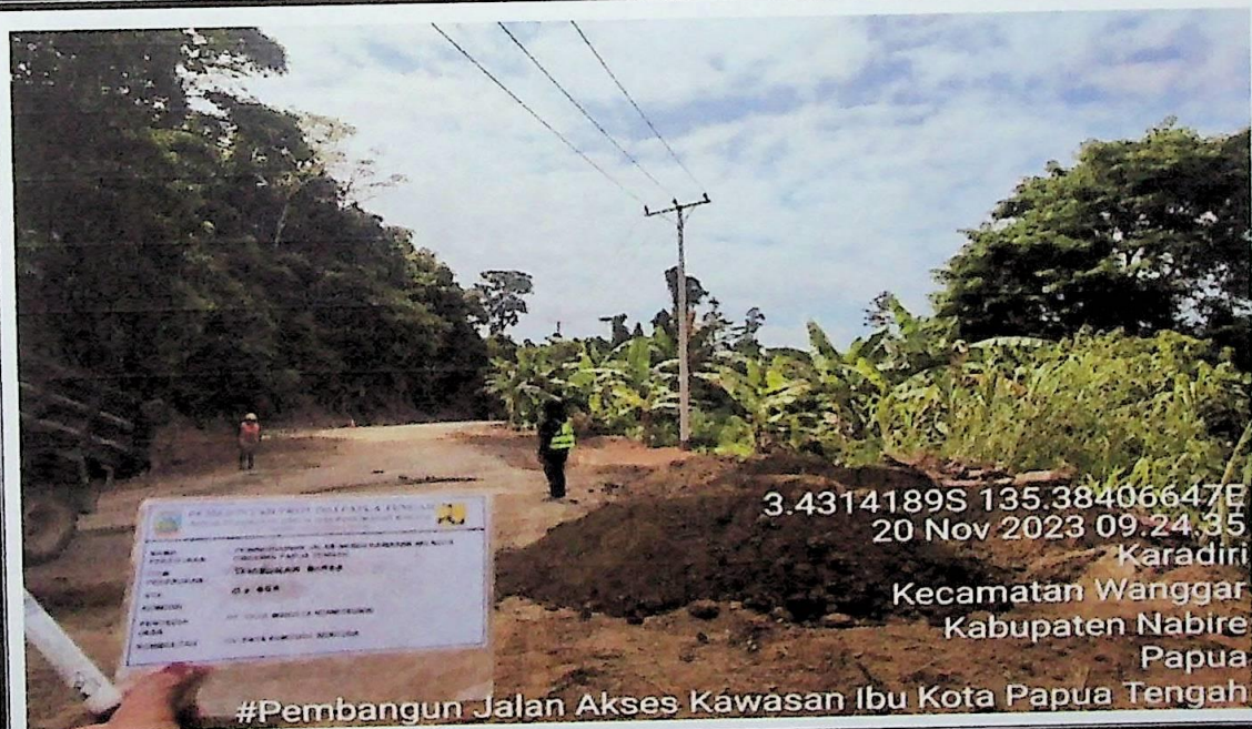
Pekerjaan galian saluran dan penyiapan badan jalan
