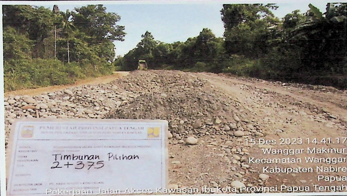
TIMBUNAN PILIHAN
